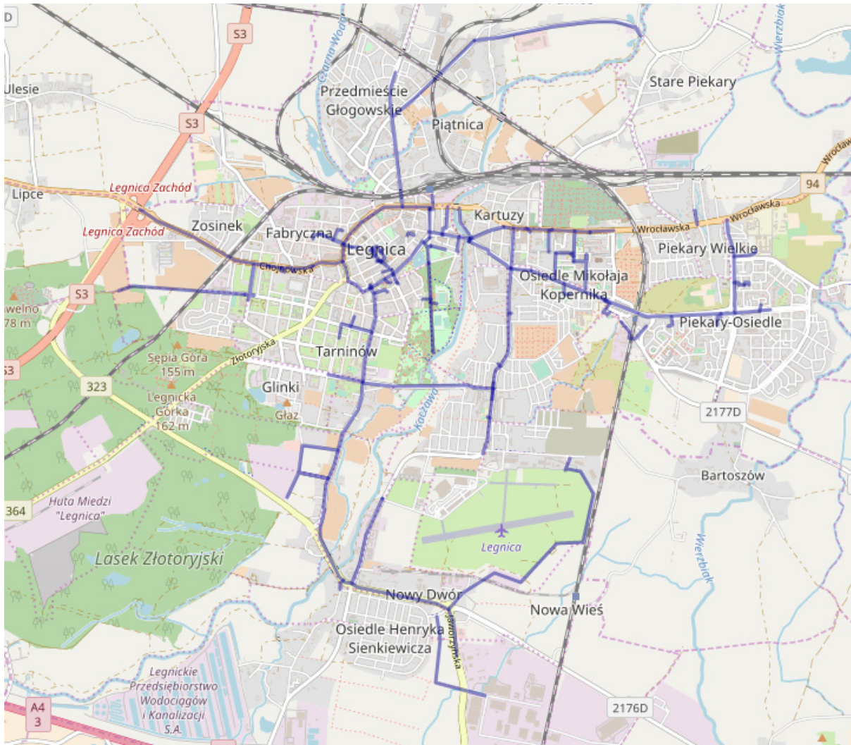
Rysunek – Mapa kanalizacji teletechnicznej LEGMAN
